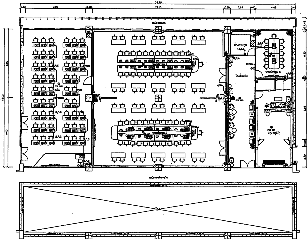
ผังเต้ารับไฟฟ้า เต้ารับโทรศัพท์ และเต้ารับคอมพิวเตอร์ ชั้น 13 1 : 75
