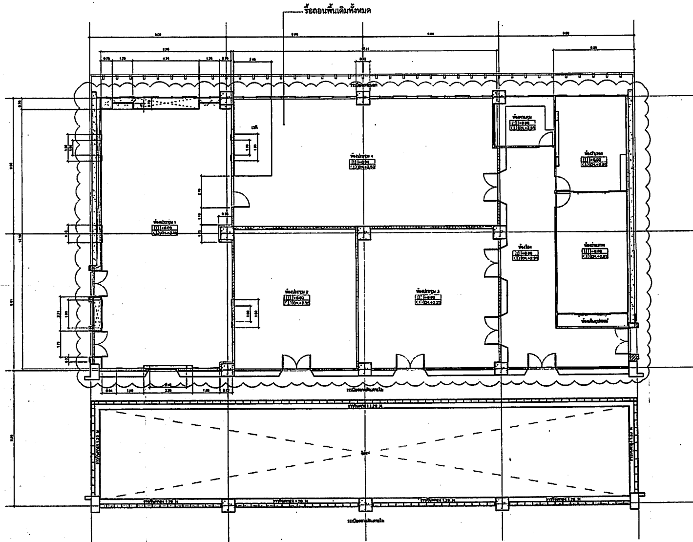
แปลนเรือคอนกรีตชั้น 13 กรมราชทัณฑ์ทางมีดง 1:75
